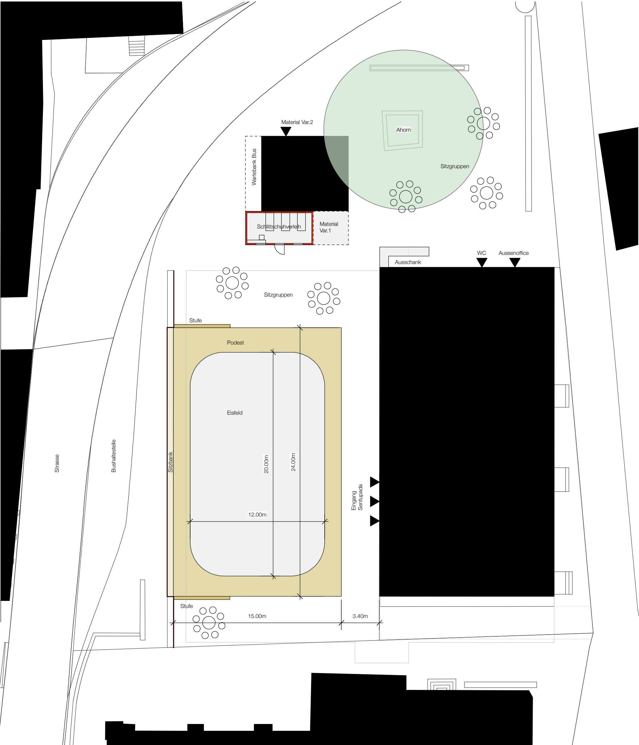
GRUNDRISS M 1:200
