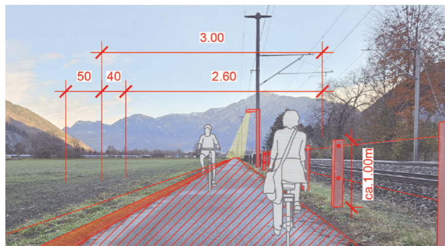
Die Region Imboden plant eine neue Veloschnellroute durchs Dorf. Eine Gesamtbreite von 3.5 Metern macht die Route sicher und bietet viel Platz für Velopendler.
